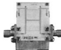
移相器回路基板
