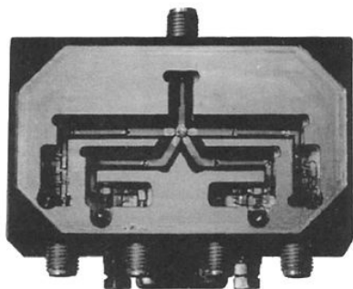
CバンドダイオードスイッチSP4T
