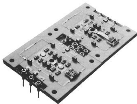
UHF帯プログラマブルアッテネータ
